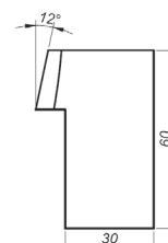
12° Spezielle Schneidplatte Höhe 60 mm Produkt-Code: NOZ-000086
