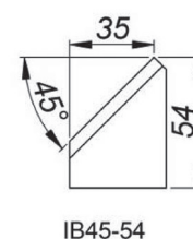
45° Innenschneidplatte für Anfasen, Höhe 54 mm [IB45/54] Produkt-Code: NOZ-000026
