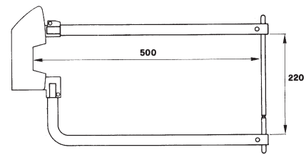
Art. 7509 Art. 7523 \varnothing 10 ▲
